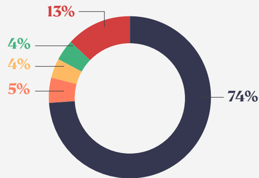
Desglose de las emisiones de GEI de alcance 1 y 2 por grupo de negocio
