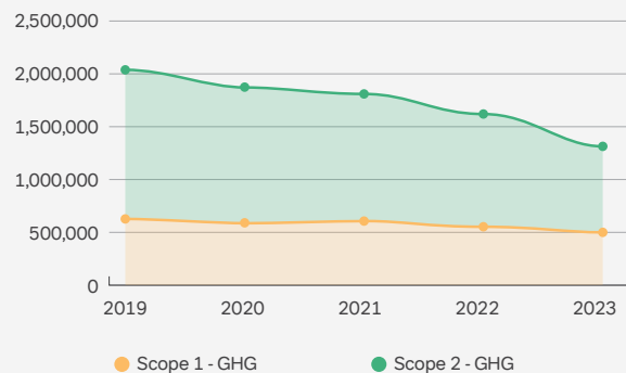
Emisiones de alcance 1 y 2 (CO 2 e total) ✓
